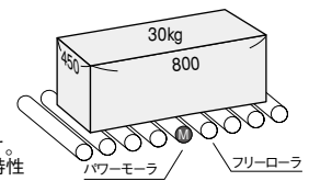
3相200V/50Hz
