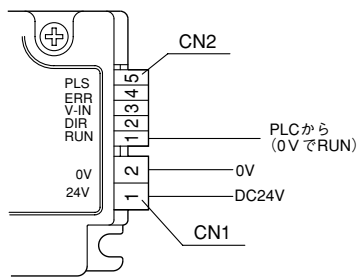
CB-016N6 配線詳細
